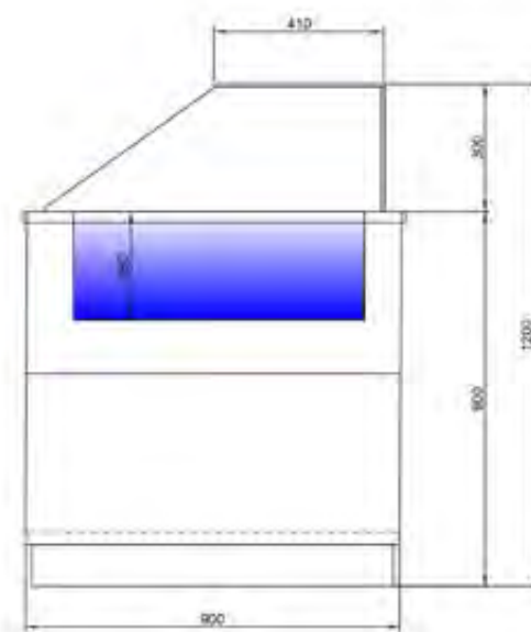
VITRINA VERSALLES CUBA CONGELACIÓN
